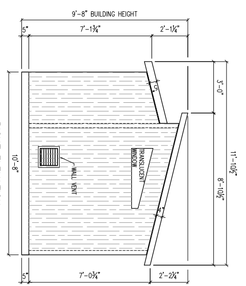
RIGHT ELEVATION
