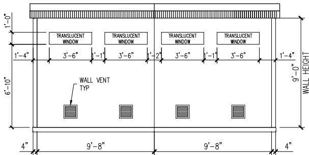
RIGHT ELEVATION
